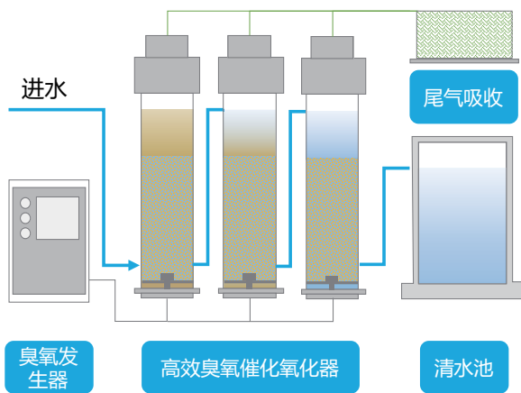
臭氧催化氧化工艺流程图
